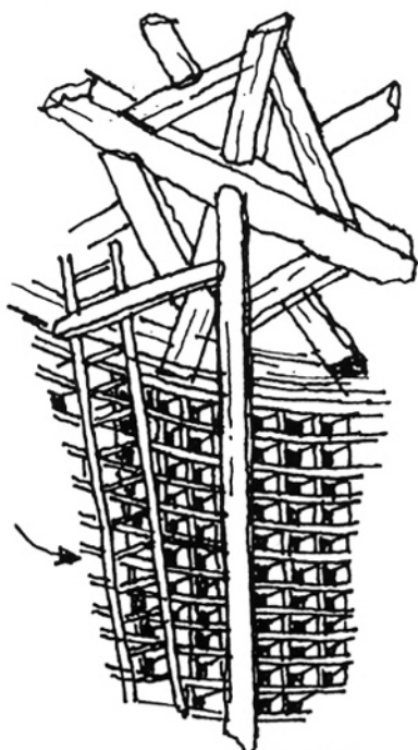
ESCALIER PIVOTANT POUR ACCEDER AUX BOULINS (CASES)
