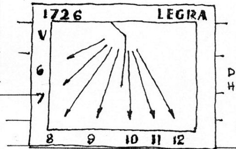
AUXONNE (21) CADRAN DECLINANT VERS LE SUD-OUEST D'ENVIRON 30° IL PEUT ETRE ECLAIRE DE 8H DU MATIN A 7H DU SOIR VERTICAL.
