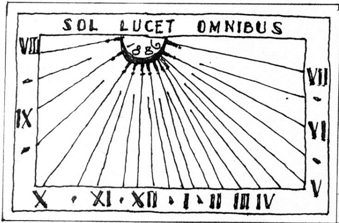
AUXONNE (21) CADRAN DECLINANT VERS LE SUD-OUEST D'ENVIRON 30° IL PEUT ETRE ECLAIRE DE 8H DU MATIN A 7H DU SOIR VERTICAL.
