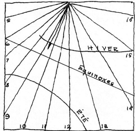
CADRAN DECLINANT DE 30° VERS L'EST ▶
